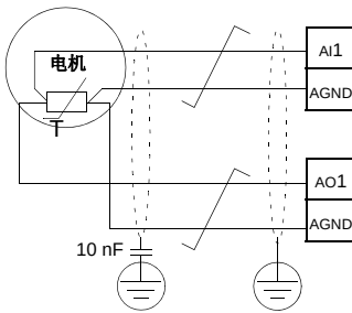
一个传感器
