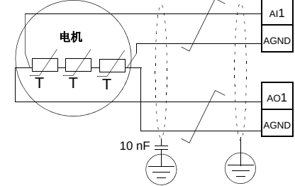
三个传感器
