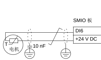
热敏电阻 (0)
