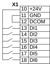
PNP 接线 (发送型)
