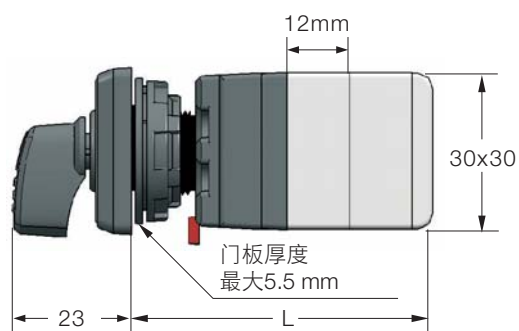
卡扣安装
