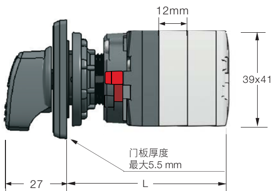
卡扣安装
